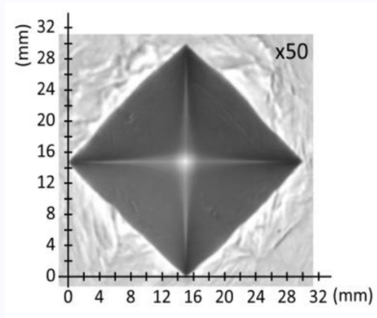
Figure 1: Huella Vickers ampliada cincuenta veces, con una diagonal de 30 mm en la escala de la imagen.
